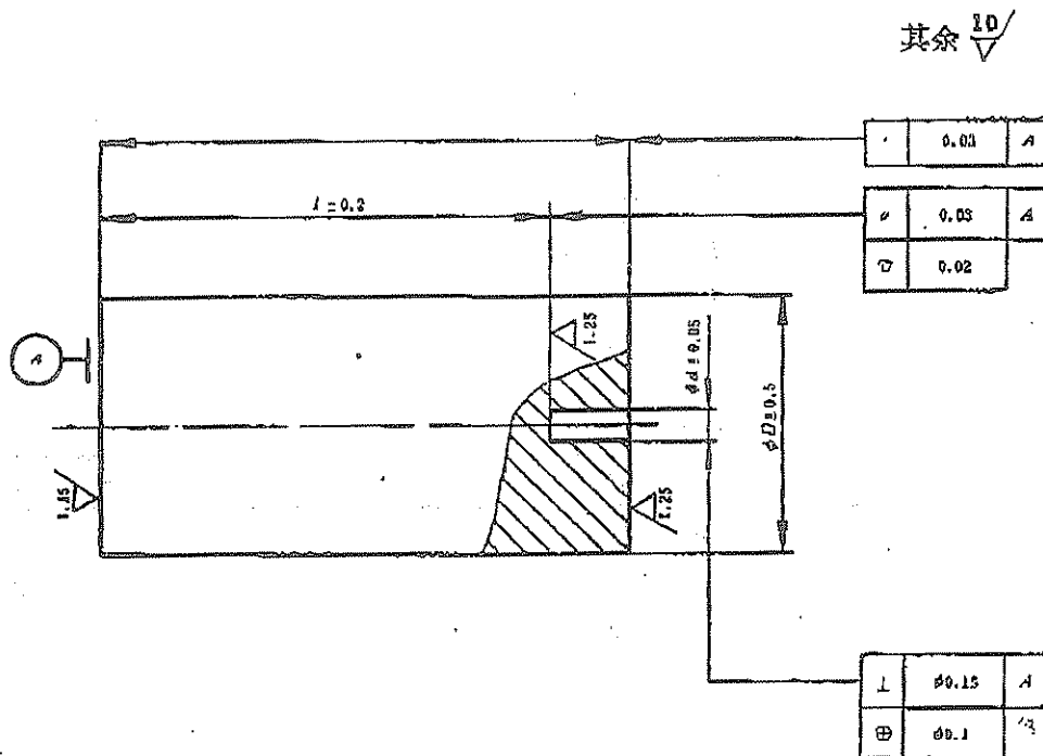
ZGZ系列对比试块
