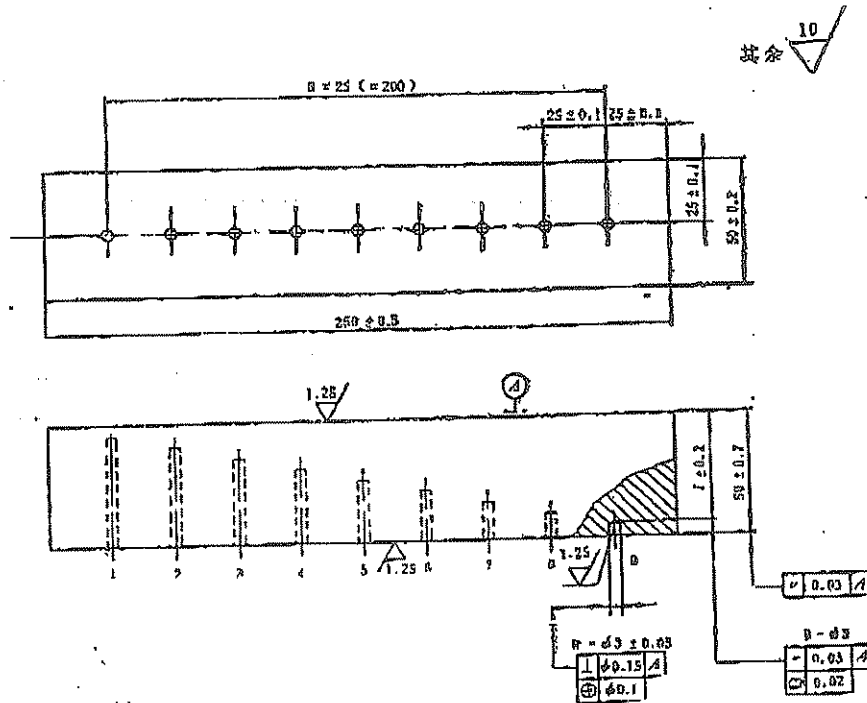
ZGS 对比试块
